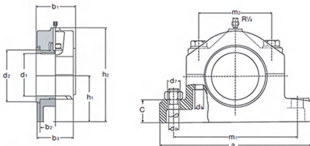
DIN 505 L 系列 DIN 505 L SERIES
